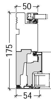
V1: PLU31-30L30 V3: PLU31-30L30 (mirr.)
