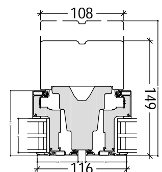
L2: PLU20-11L44
