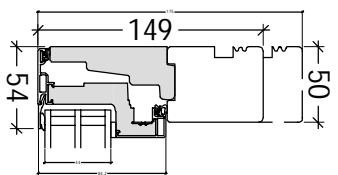
V1/V4: PLU20-30L44 V3/V5: PLU20-30L44(mirr.)
