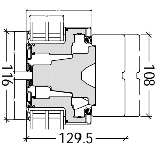
L2: PLU20-12L44
