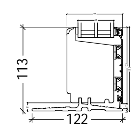
L4: FRAic23-12L48
