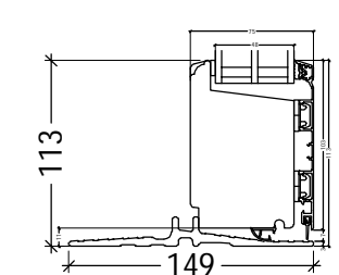
L4: FRAic23-15L48
