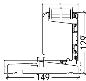
L4: FRAic23-12L48
