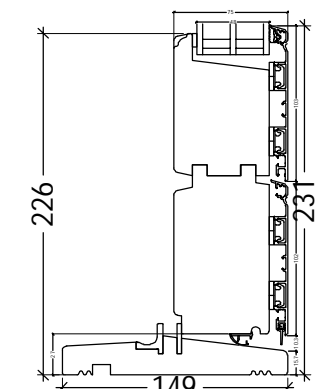
L4: FRAic23-16L48
